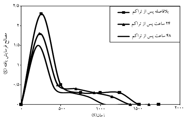
شکل ۲۸. منحنی میزان فرسایش یافته در برابر زمان برای زمان‌های مختلف تراکم.
