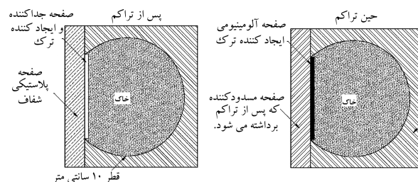
شکل ۹. مقطع عرضی دستگاه SCT در حالت‌های قبل و بعد از برداشتن صفحه‌ی آلومینیومی و شکل‌گیری ترک خوردگی.
