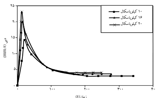
شکل ۱۷. تغییرات دبی در برابر زمان برای فشارهای مختلف در زمان کوتاه.
