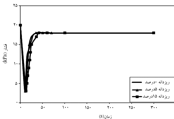
شکل ۲۲. منحنی فشار در برابر زمان برای درصدهای ریزدانه‌ی مختلف.
