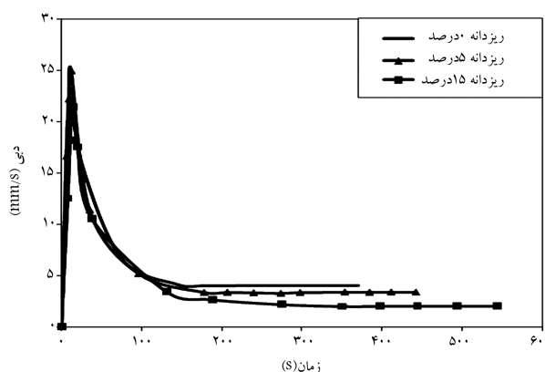
شکل ۲۱. منحنی دبی در برابر زمان برای درصدهای ریزدانه‌ی مختلف.
