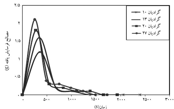
شکل ۲۷. منحنی میزان فرسایش یافته در برابر زمان برای گرادیان‌های هیدرولیکی مختلف.
