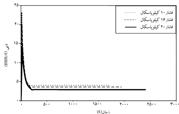
شکل ۱۸. تغییرات دبی در برابر زمان برای فشارهای مختلف در زمان طولانی.
